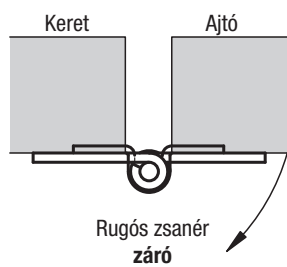
felhelyezett szerelvény:
