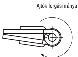
Zsanérok zárórugóval
